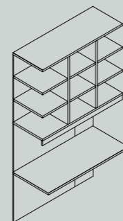
Modulo ponte libreria con scrittoio L 1480/1978 H 822/1142 P 360 Bridging unit w/bookcase and desktop W 1480/1978 H 822/1142 D 360
