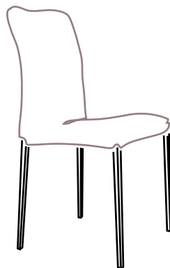
P20 Sedia con struttura metallica con tubo piramidale da 20x20-14x14 mm / Metal structure chair in pyramidal tube 20x20-14x14 mm
